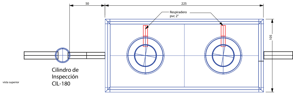
Filtro Anaeróbico de Flujo Ascendente FAFA-1600
