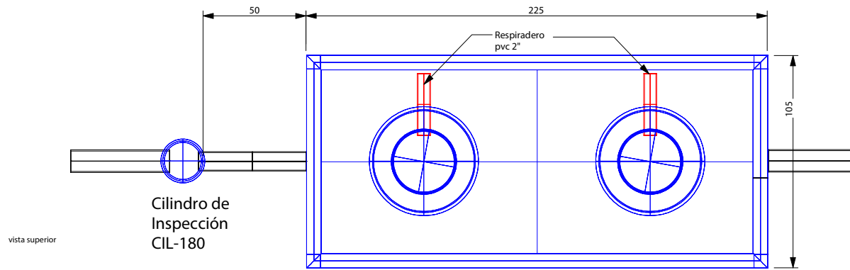
Filtro Anaeróbico de Flujo Ascendente FAFA-1600
